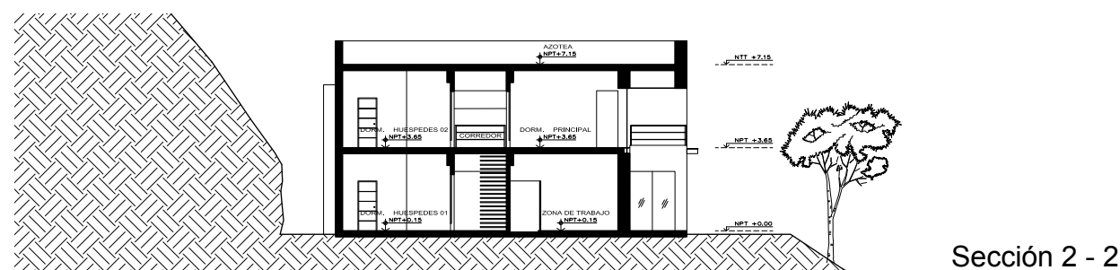
Sección 2 - 2
