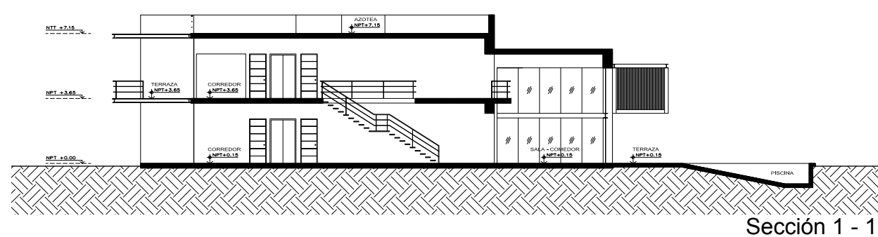
Sección 1 - 1
